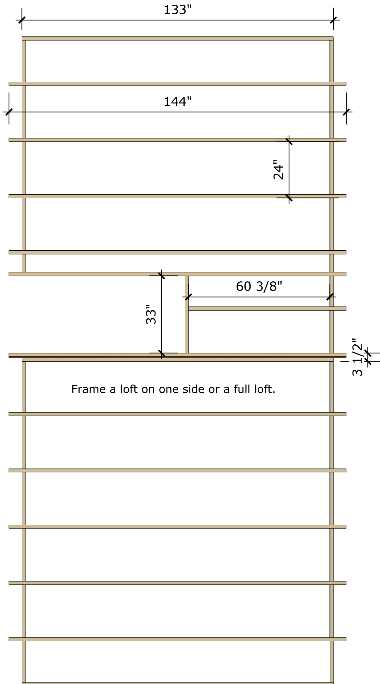
Loft Framing
